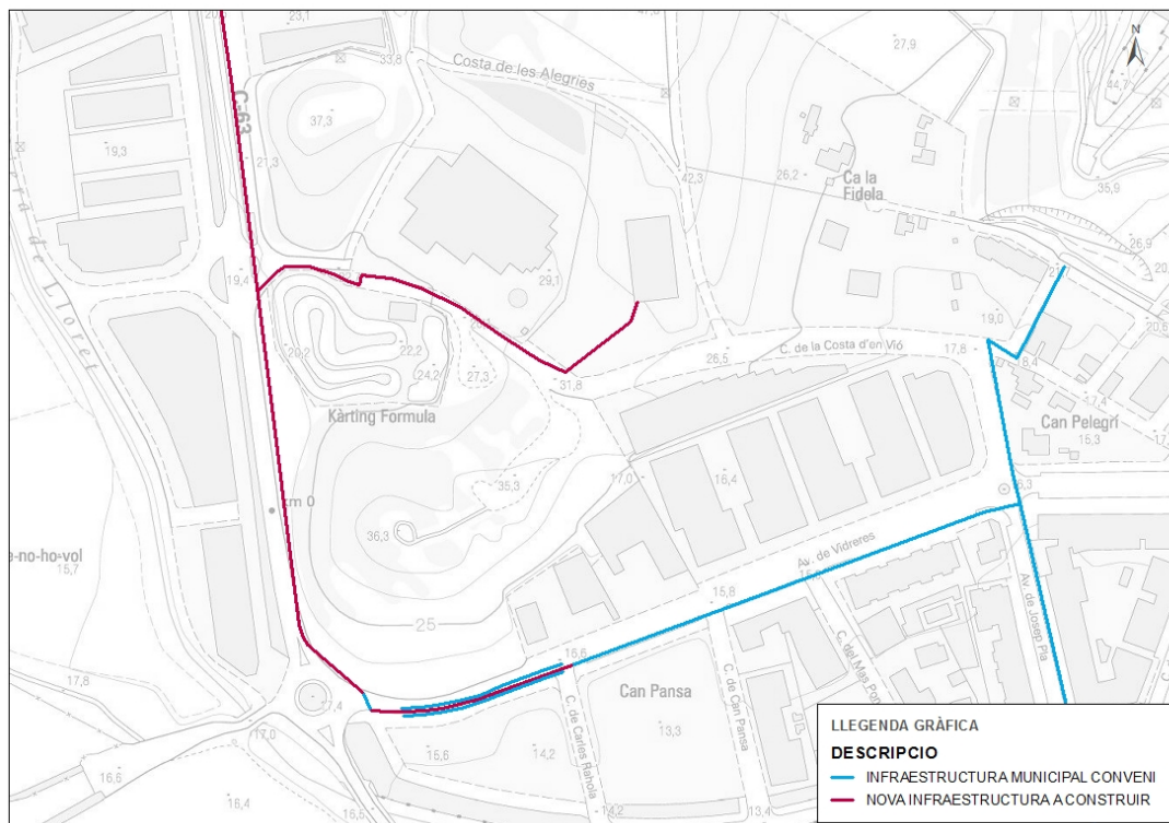
Figura 1.1 Plànol detall d'infraestructures accés Nord que són objecte del conveni al municipi de Lloret de Mar
