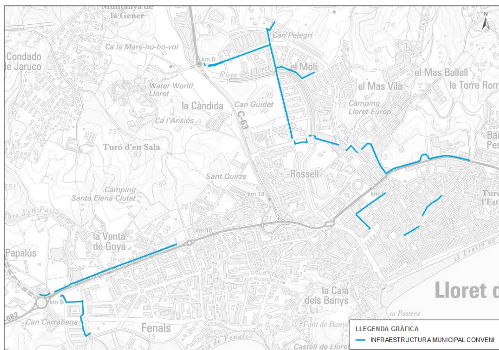
Figura 2 Plànol de la compartició d'ús de canalització municipal
