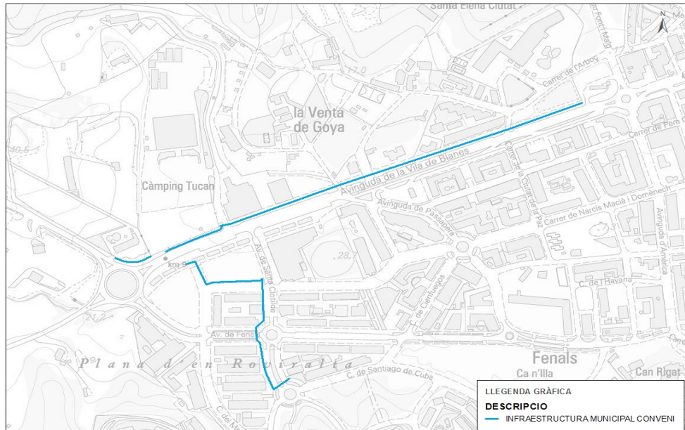
Figura 1.3 Plànol detall d'infraestructures accés oest que són objecte del conveni al municipi de Lloret de Mar
