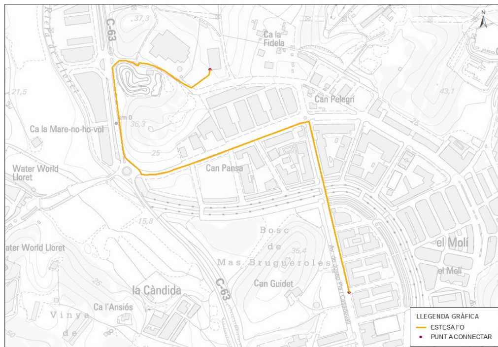
Figura 4 Plànol de la cessió d'ús de fibra òptica. Instal·lacions a realitzar pel CTTI
